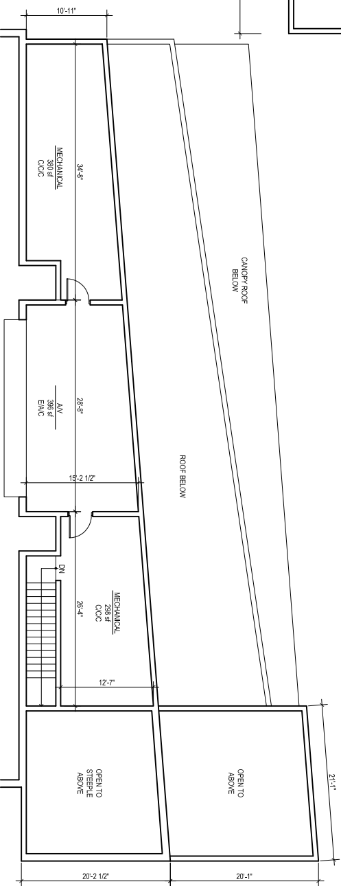
2 MEZZANINE PLAN SCALE: 1/8" = 1'-0"
